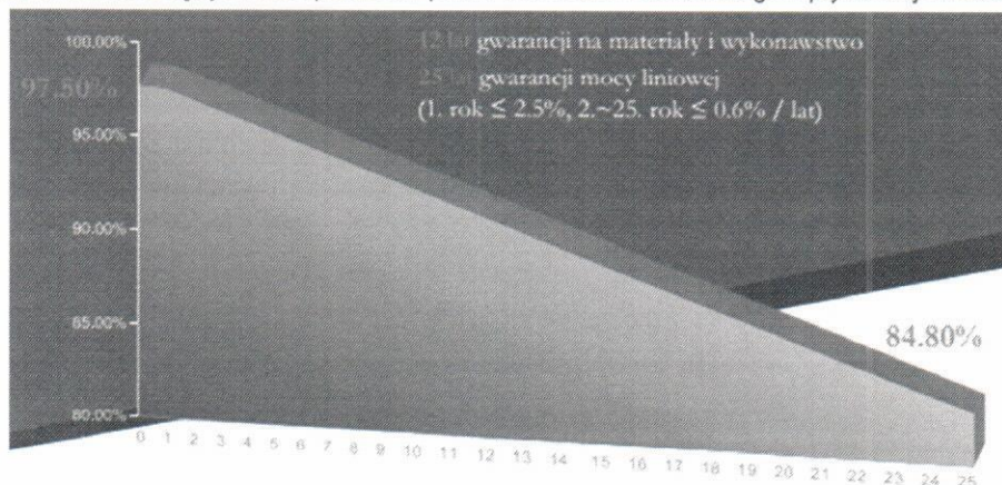
Rys. nr 1: Przykład linearyzacji charakterystyki degradacji mocy paneli fotowoltaicznych w funkcji czasu
